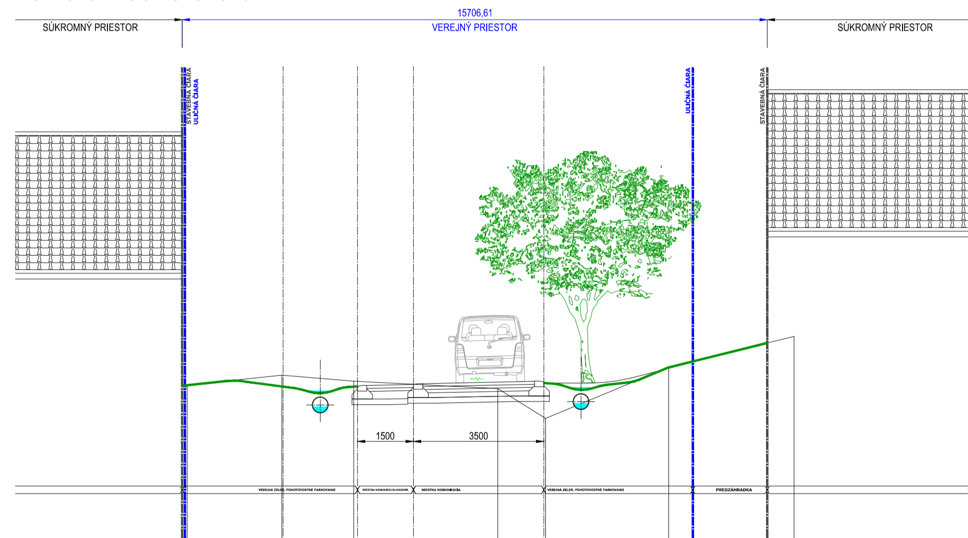
rez d-d Podhorská ul.
