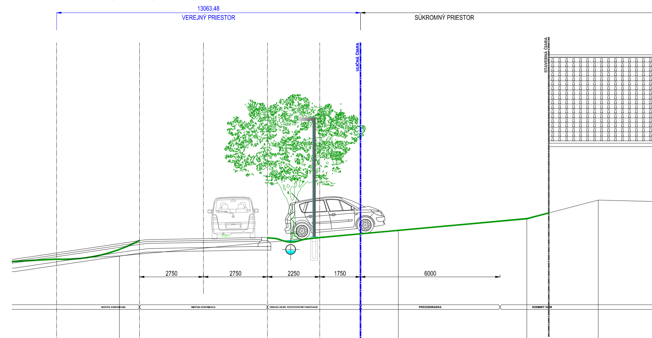
rez a-a Podhorská ul.
