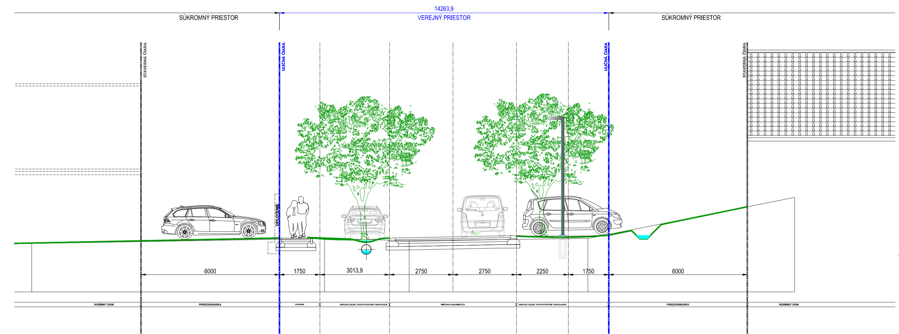
rez c-c Podhorská ul.
