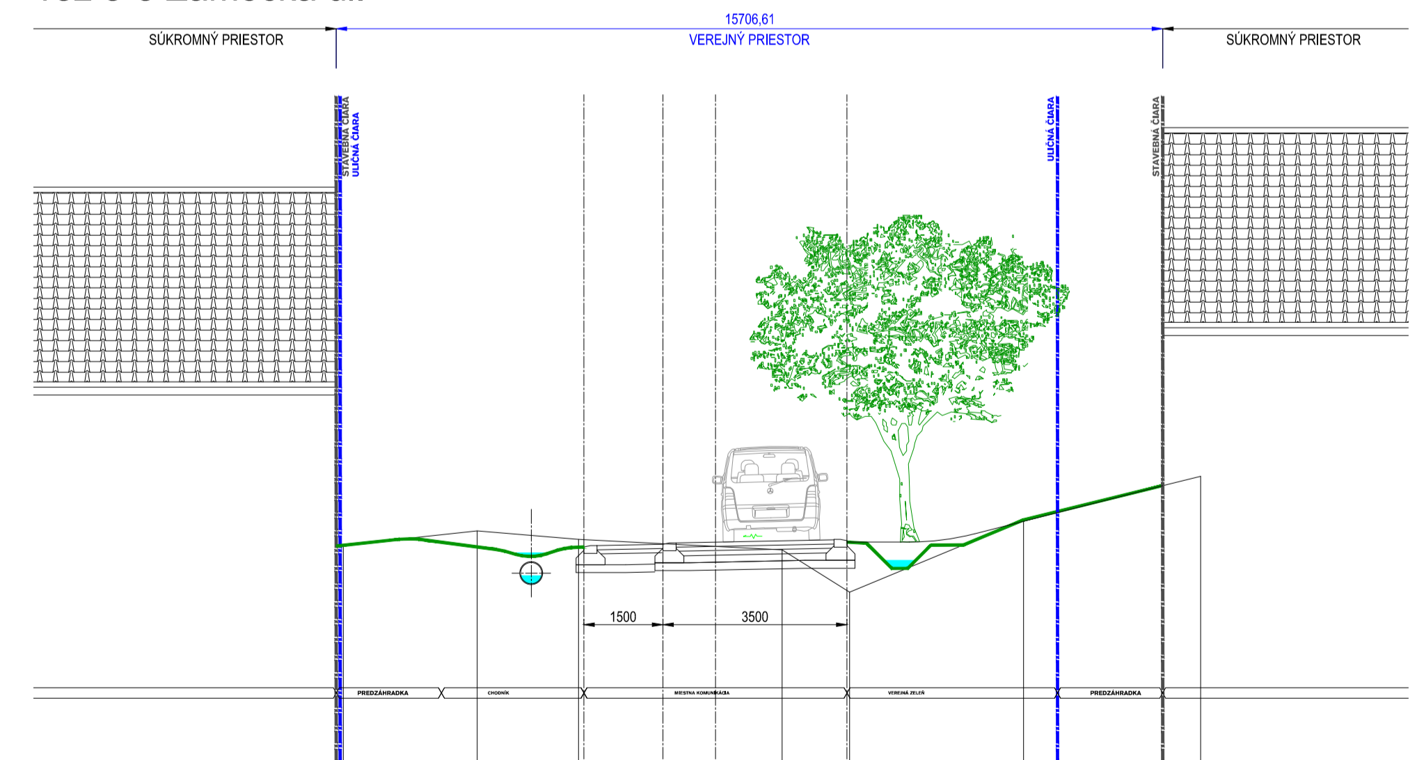
rez e-e Zámocká ul.
