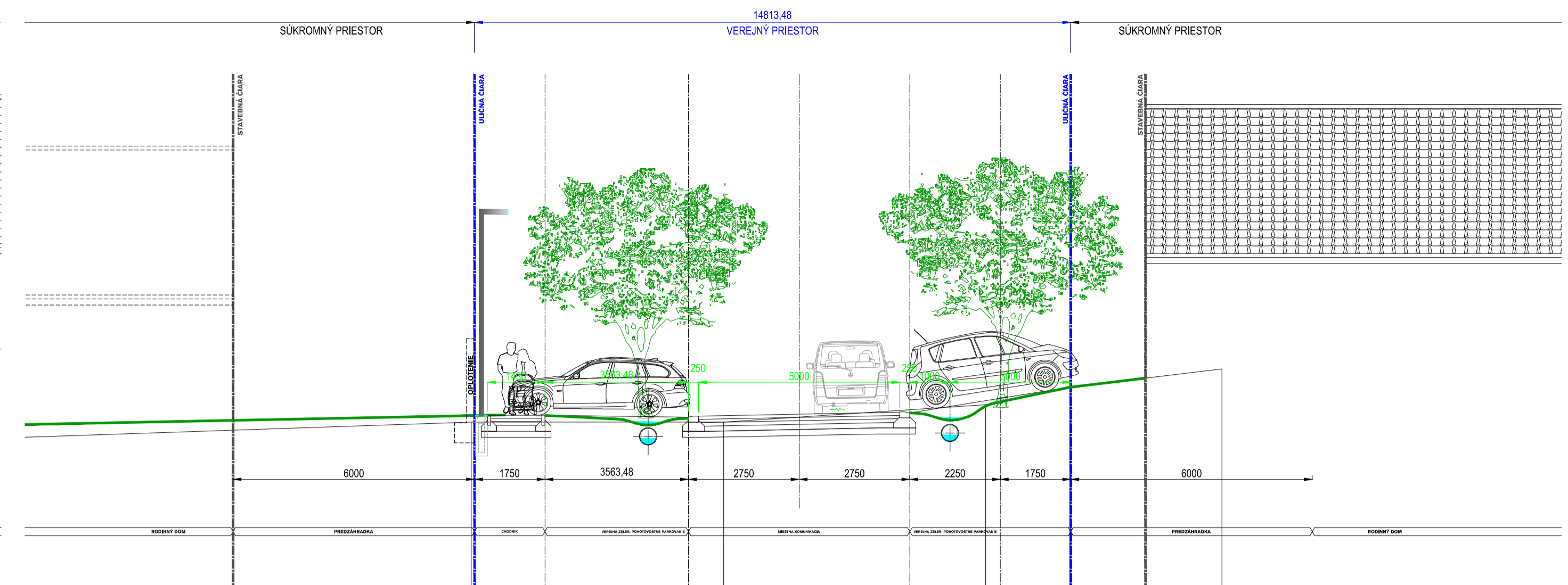
rez b-b Podhorská ul.
